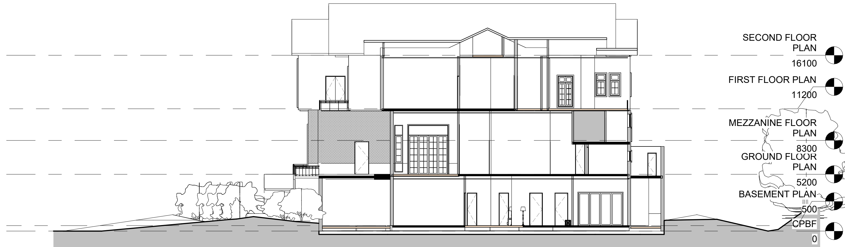
1 Section AA 1 : 200
